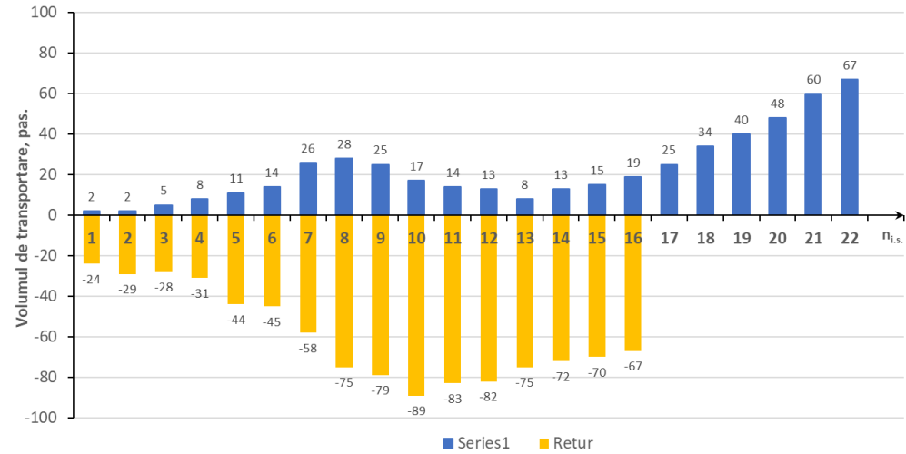
Figura 4.13 Graficul fluxului de pasageri pe ruta nr. 37 tur-retur în orele de vârf dimineața
