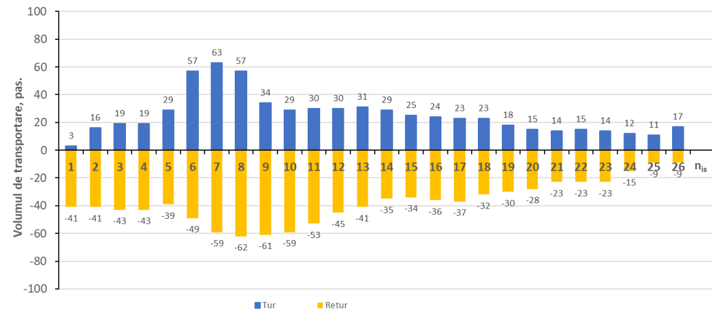
Figura 4.16 Graficul fluxului de pasageri pe ruta nr. 28 tur-retur în orele de vârf dimineața
