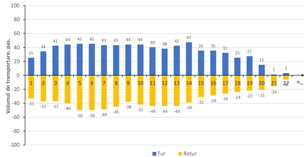
Figura 4.4 Graficul fluxului de pasageri pe ruta nr. 2 tur-retur în orele de vârf dimineața
