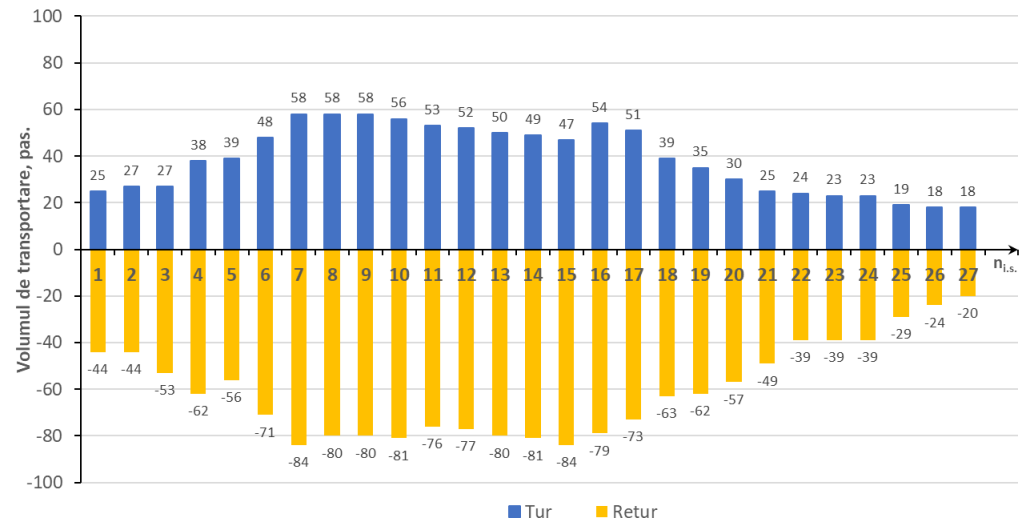
Figura 4.10 Graficul fluxului de pasageri pe ruta nr. 48 tur-retur în orele de vârf dimineața
