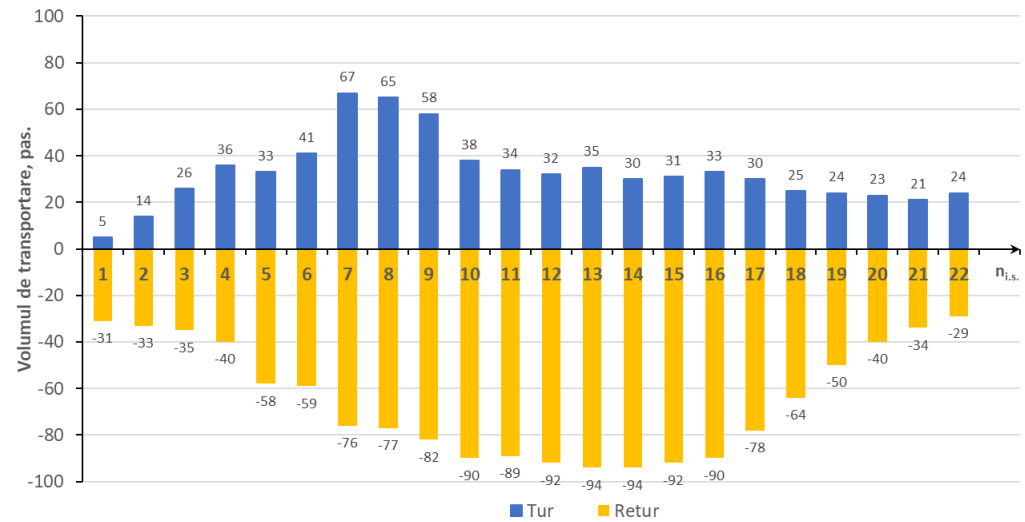
Figura 4.7 Graficul fluxului de pasageri pe ruta nr. 47 tur-retur în orele de vârf dimineața
