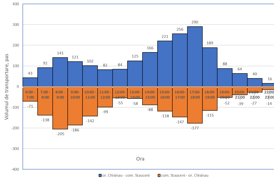
Figura 4.12 Volumele orare de călători pe ruta nr. 37 or. Chișinău–or. Stăuceni
