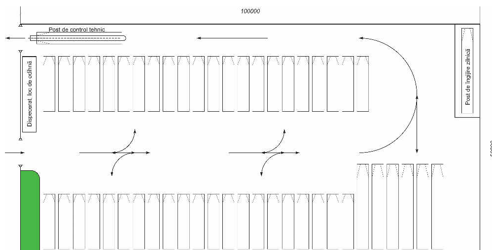
Figura 4.23 Proiect de teren tehnologic în zona stației „Cercul”
