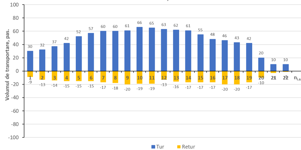
Figura 4.5 Graficul fluxului de pasageri pe ruta nr. 2 tur-retur în orele de vârf seara
