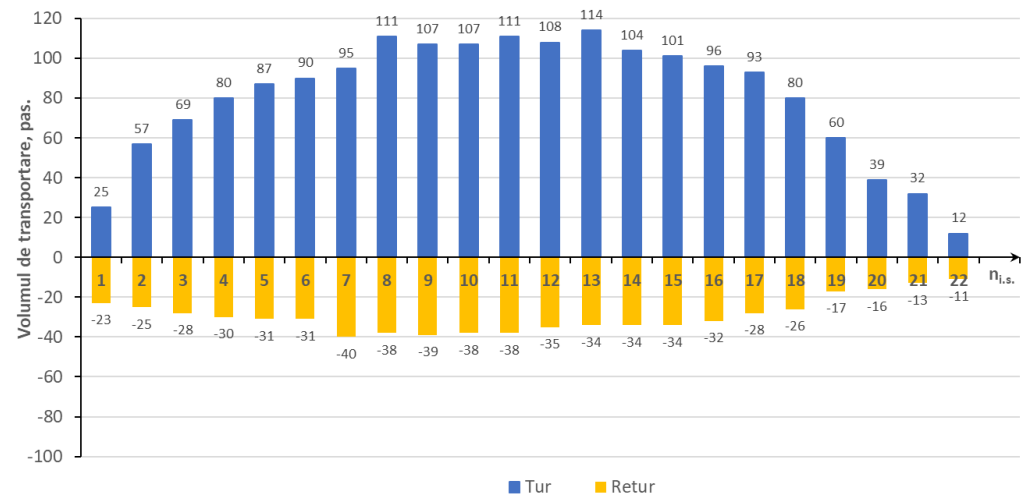
Figura 4.8 Graficul fluxului de pasageri pe ruta nr. 47 tur-retur în orele de vârf seara
