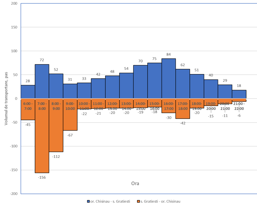
Figura 4.18 Volumele orare de călători pe ruta nr. 10 or. Chișinău–s. Grățiești
