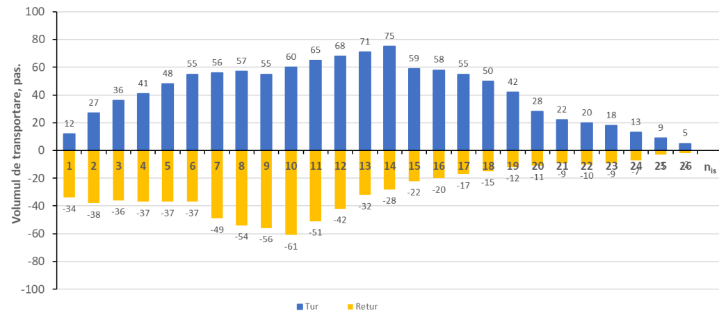
Figura 4.17 Graficul fluxului de pasageri pe ruta nr. 28 tur-retur în orele de vârf seara
