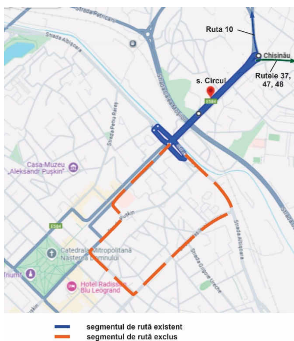
Figura 4.21 Modificările propuse pentru rutele suburbane nr. 10, 37, 47, 48, din zona stației „Cercul”
