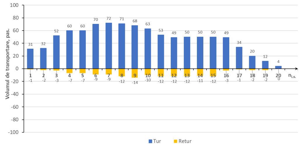
Figura 4.20 Graficul fluxului de pasageri pe ruta nr. 10 tur-retur în orele de vârf seara
