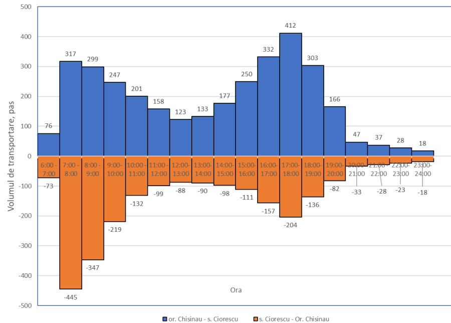
Figura 4.6 Volumele orare de călători pe ruta nr. 47 or. Chișinău–s. Ciorescu
