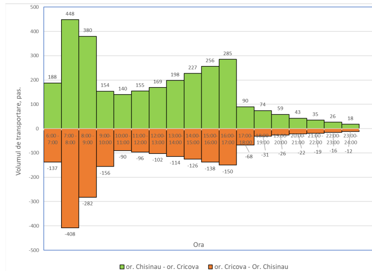
Figura 4.3 Volumele orare de călători pe ruta nr. 2 or. Chișinău–or. Cricova
