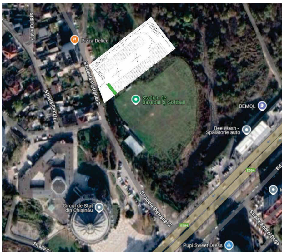
Figura 4.22 Amplasarea terenului tehnologic în zona stației „Cercul”
