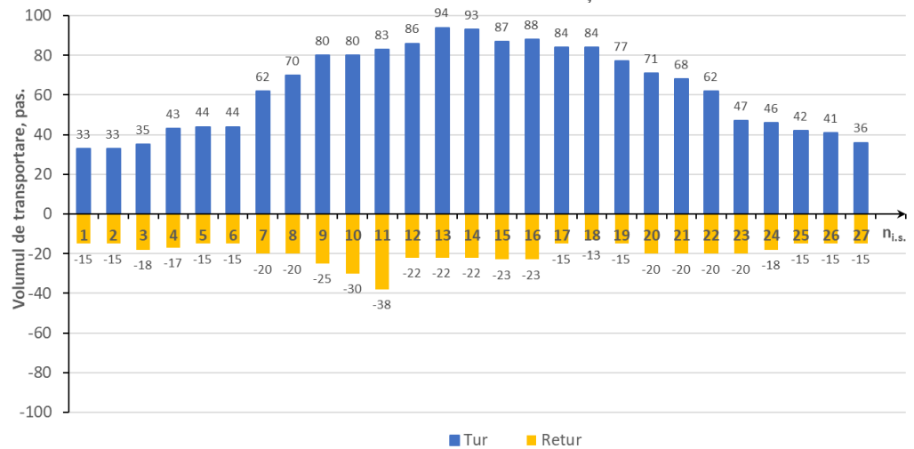
Figura 4.11 Graficul fluxului de pasageri pe ruta nr. 48 tur-retur în orele de vârf seara
