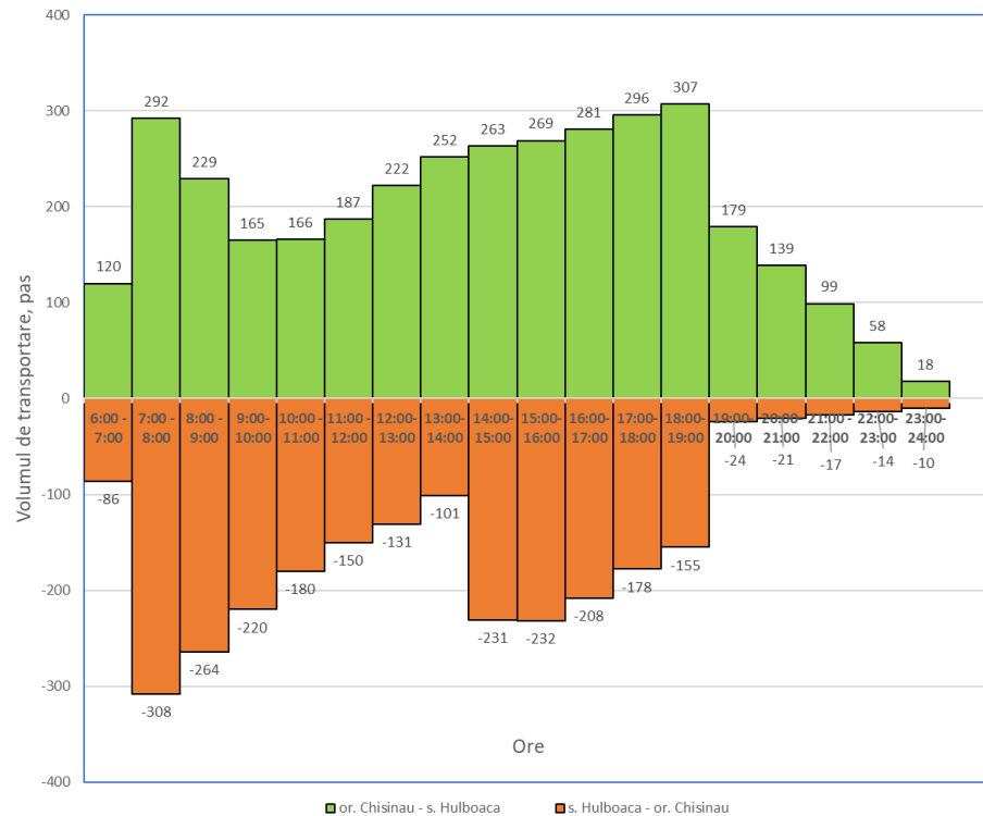
Figura 4.15 Volumele orare de călători pe ruta nr. 28 or. Chișinău–s. Hulboaca
